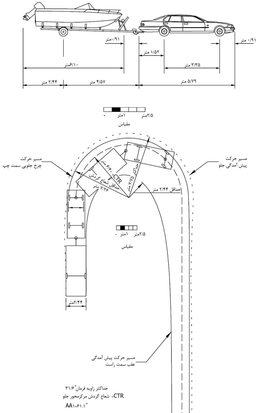
شکل ۴-۱- حداقل مسیر گردشی برای وسیله طرح سواری با یدک قایق
