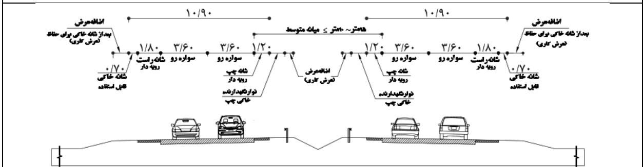
A۵- راه شریانی جداشده چهار خطه با میانگین متوسط
