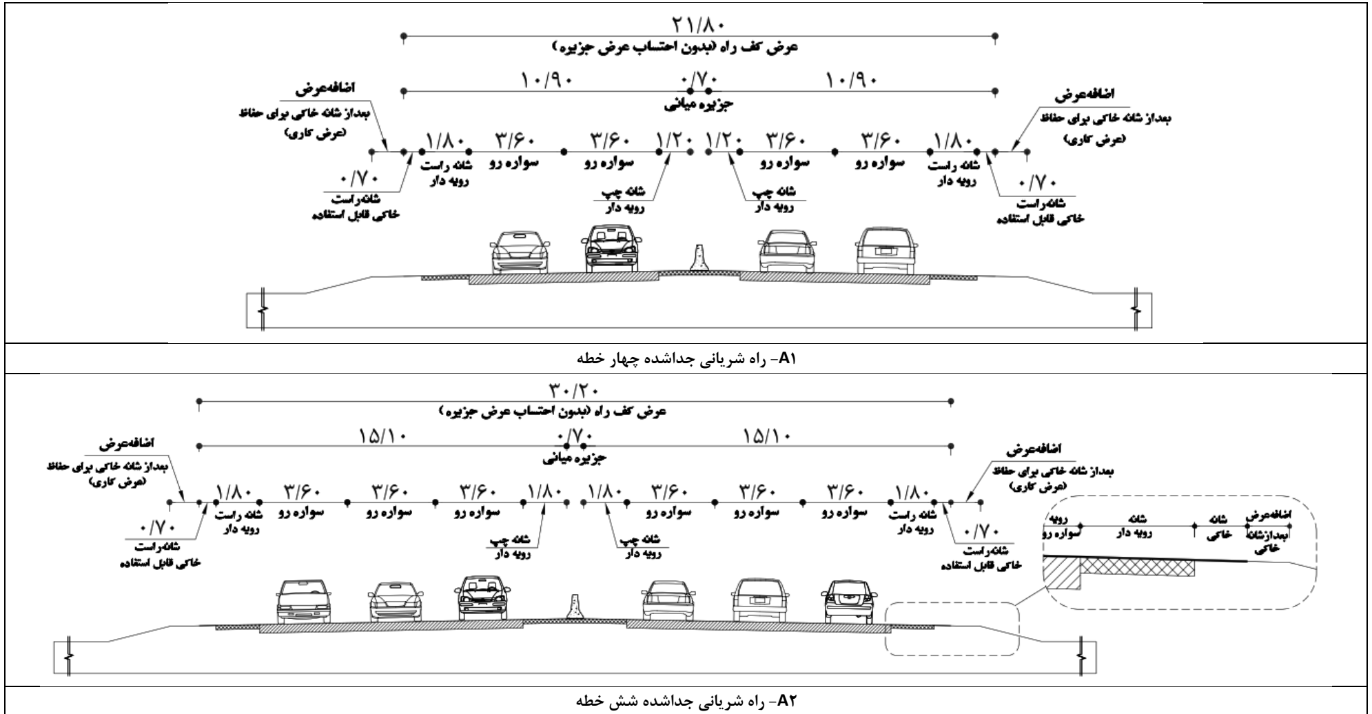
مقاطع نمونه راه شریانی
